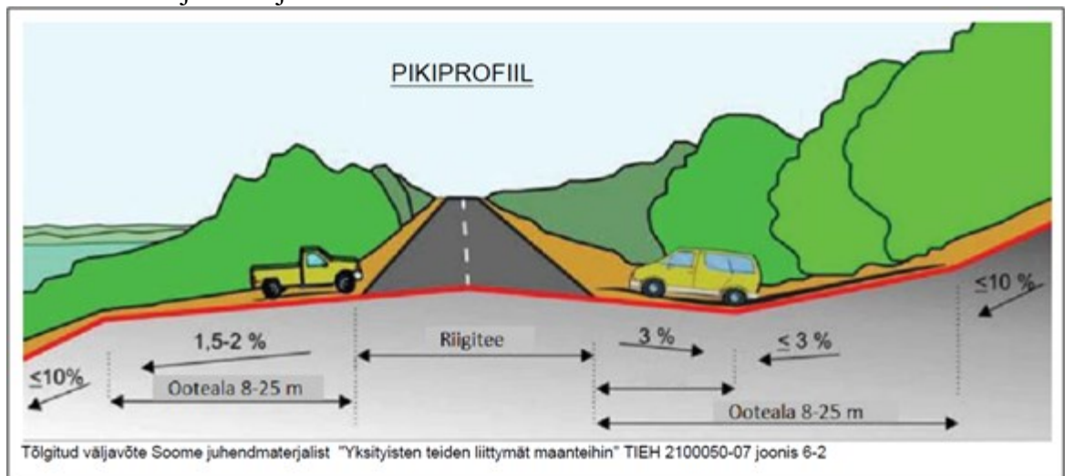
Joonis 2. Ristumiskoha pikikallate kujundamine
